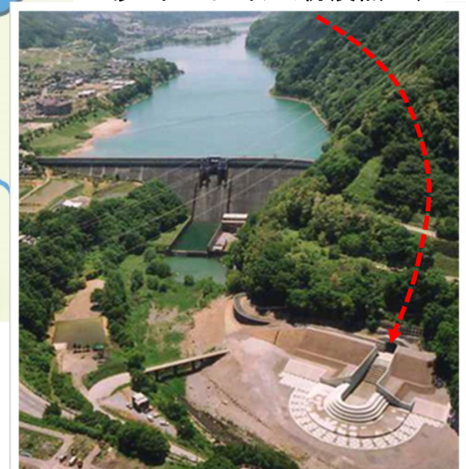
土砂バイパストンネルの例(美和ダム)
