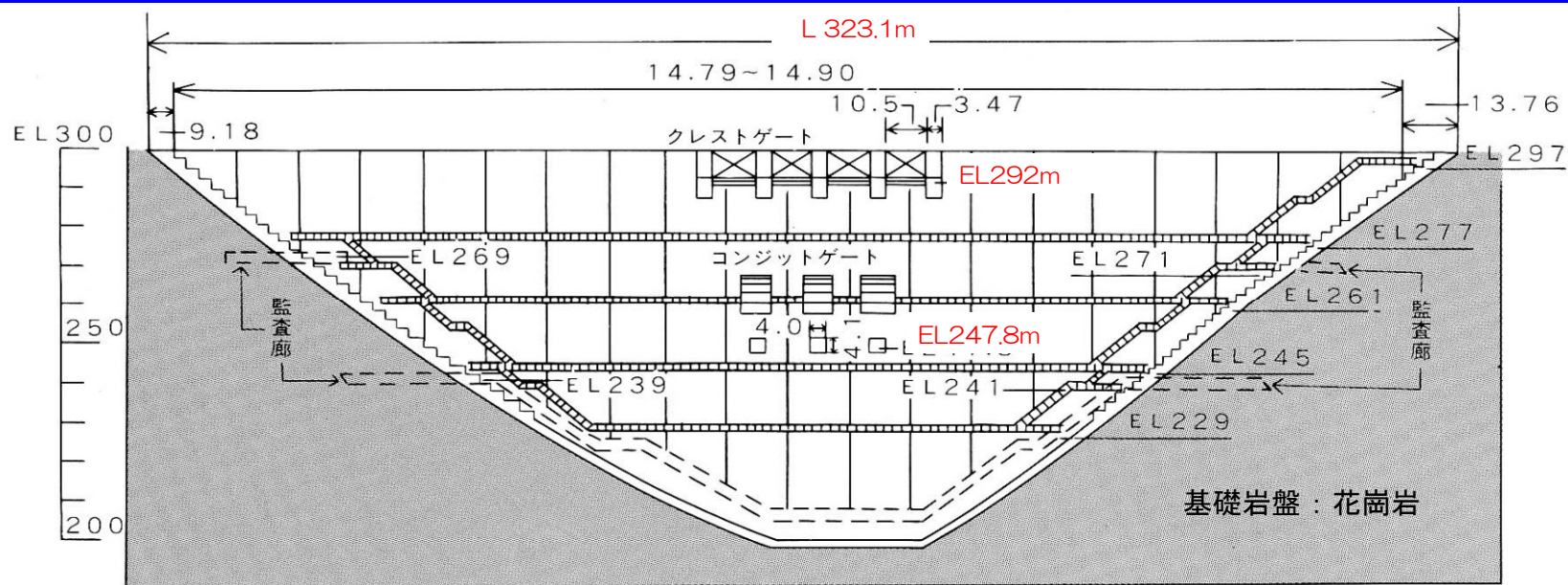
ダム下流面図
