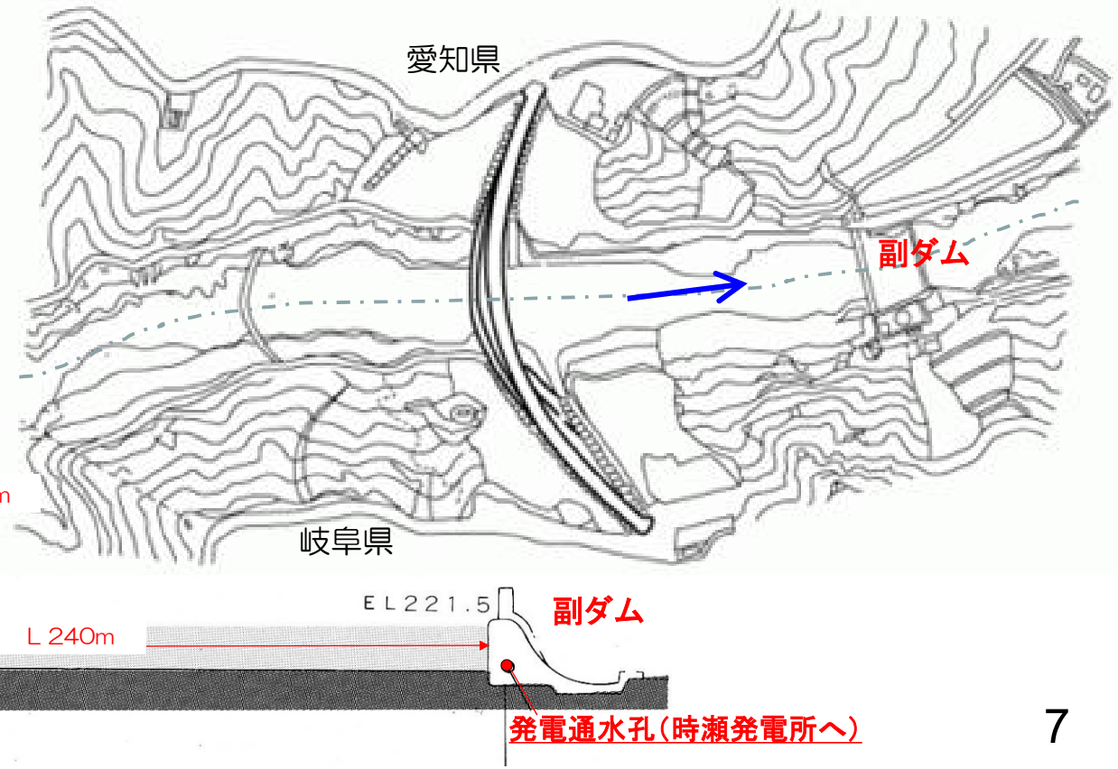
ダム平面図
