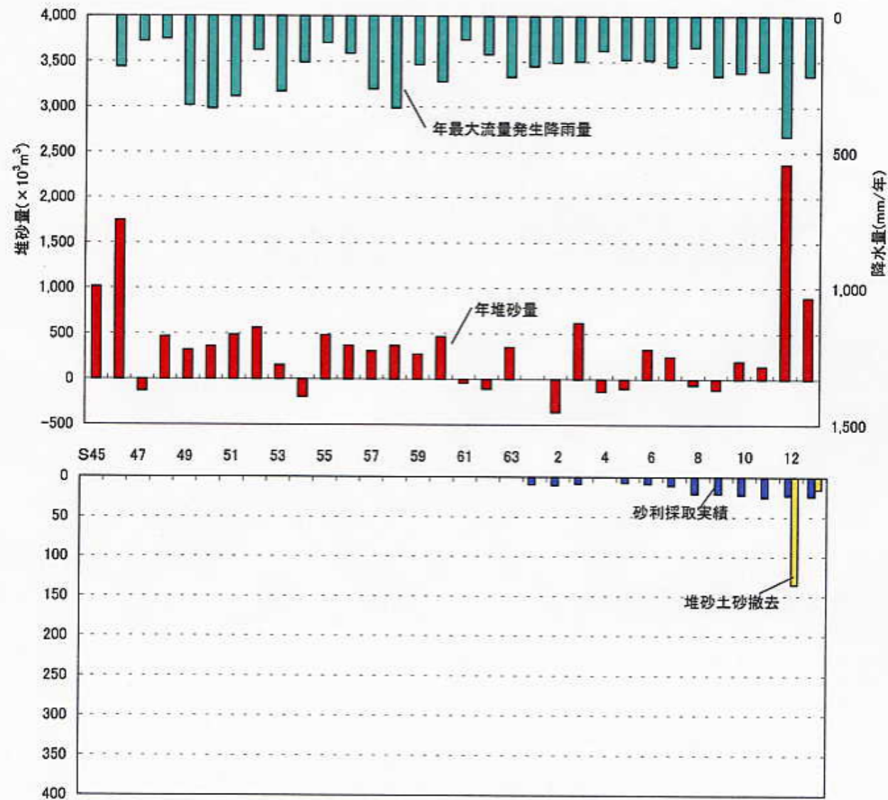
○矢作ダム堆砂量等の経年変化
