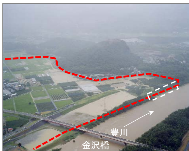
洪水時の金沢霞堤地区（平成15年8月）
