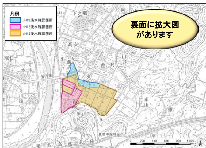
金沢霞堤地区の近年の浸水実績
