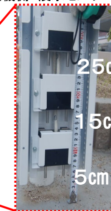
<浸水センサ3段>
