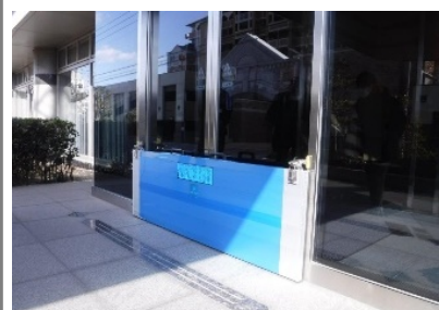
パネル型簡易止水版
