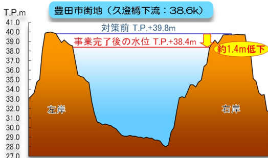
●対策による水位低下効果（横断面）
