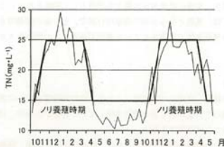
図 3.2.5 浄化センターの栄養塩管理運転による排出水のTN濃度の変化(目標イメージ)
