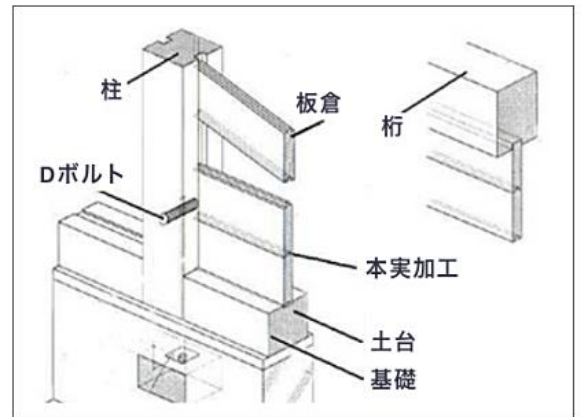
板倉構法模式図。釘を使わず、柱と柱の間に板を落とし込む（東海林建築設計事務所HPより）
