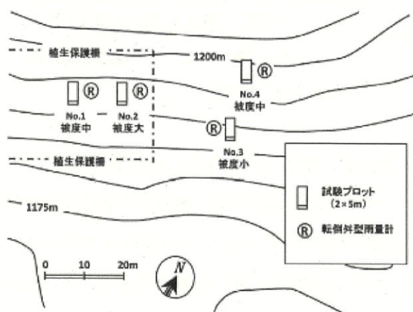
図 試験プロット配置図
