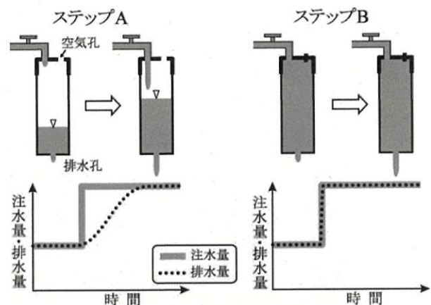
図 注水量変化の排水量変化への伝わり方
