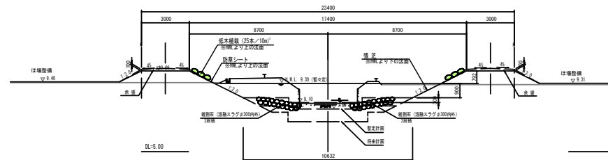
標準断面図
