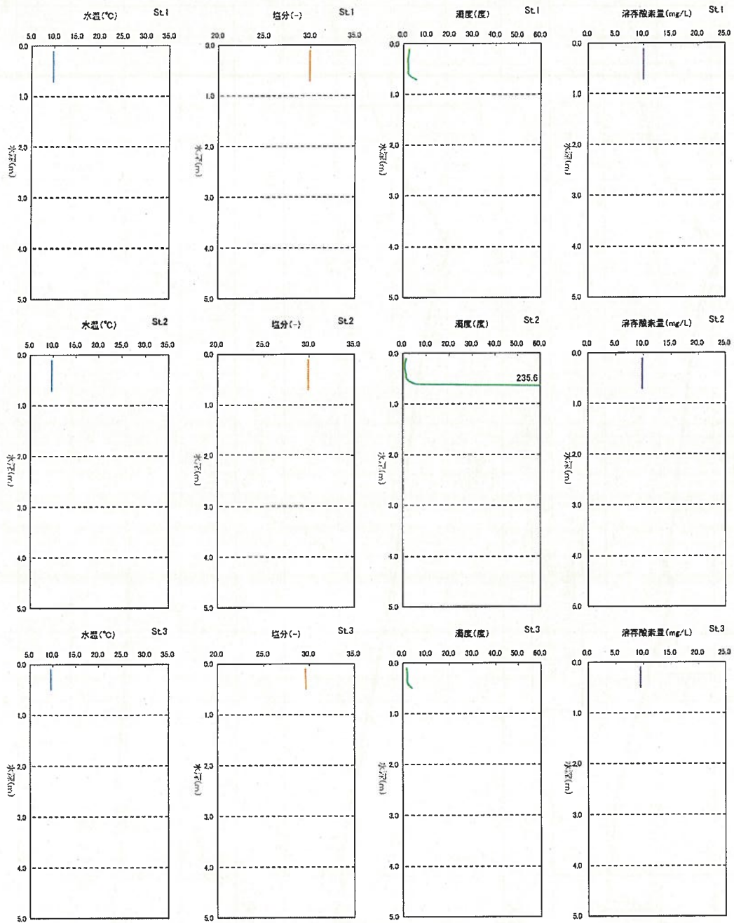
図 11(1) 水質調査結果 (冬季)
