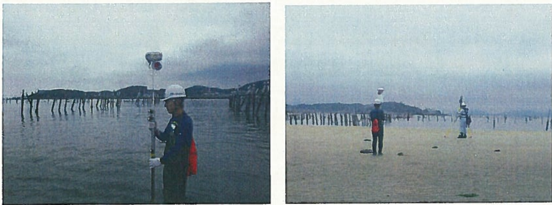
図 3 地形調査（深浅測量）の実施状況
