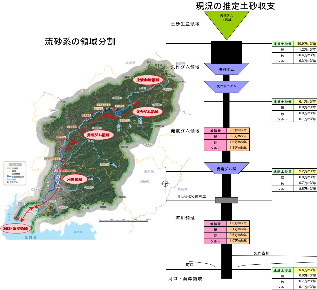
河床変動計算による推定値
