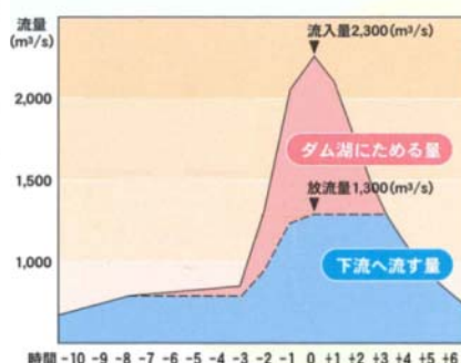
矢作ダム洪水調節計画
