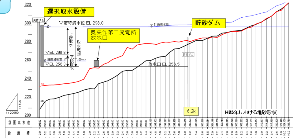
貯水池縦断面図(H25)
