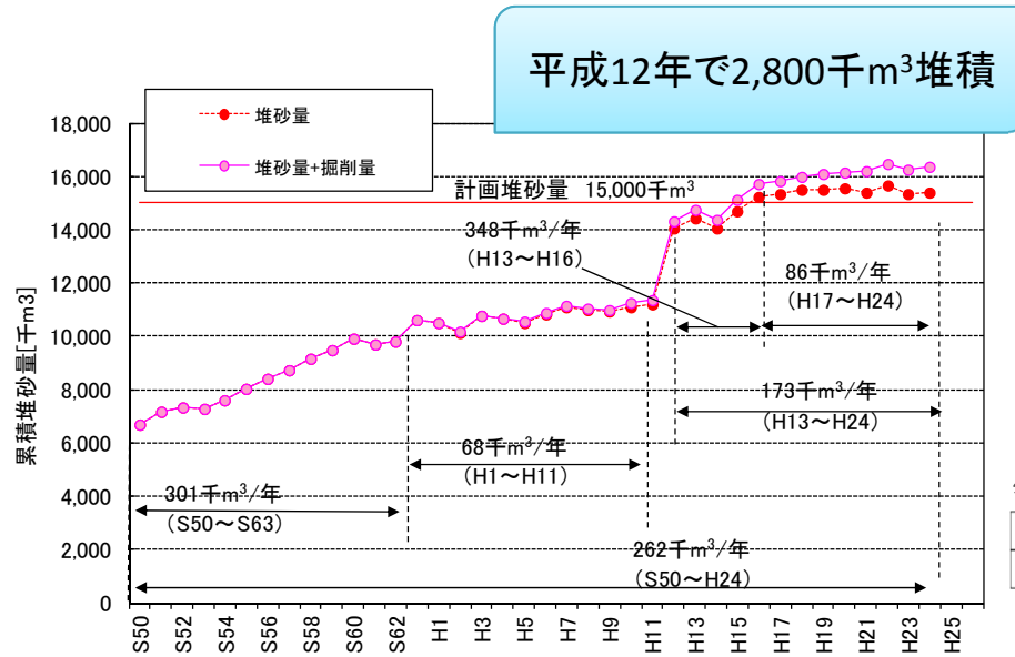
矢作ダム堆砂実績図
