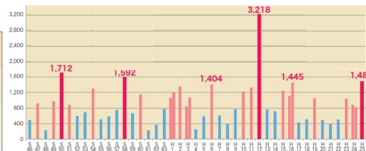
矢作ダム洪水発生状況 3
