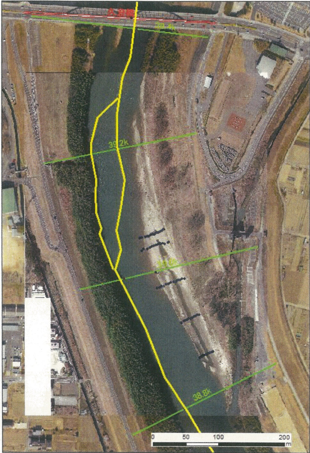
図-3 縦断計測測線と、横断の位置図
