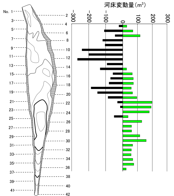
図 7 工事後から 2009 年 4 月の河床変動量
