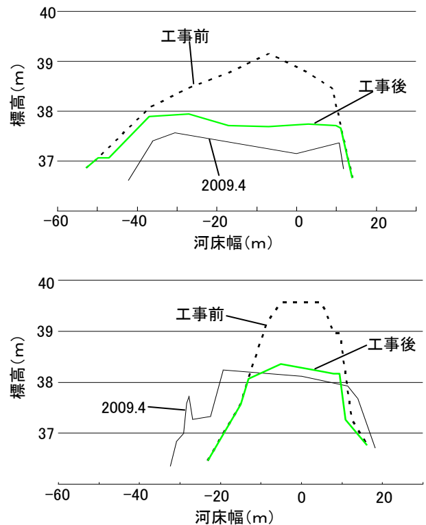
図 8 侵食が最も大きかった No. 12(上)と堆積が最も大きかった No. 22(下)
