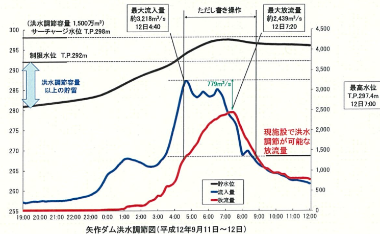
矢作ダム洪水調節図 (平成12年9月11～12日) 平成12年9月洪水
