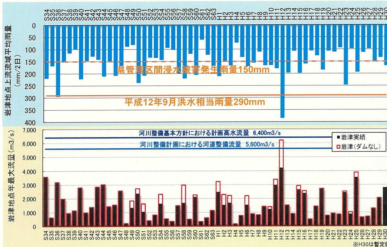
矢作川(岩津地点)の年最大流量および流域平均雨量(年最大2日雨量)
