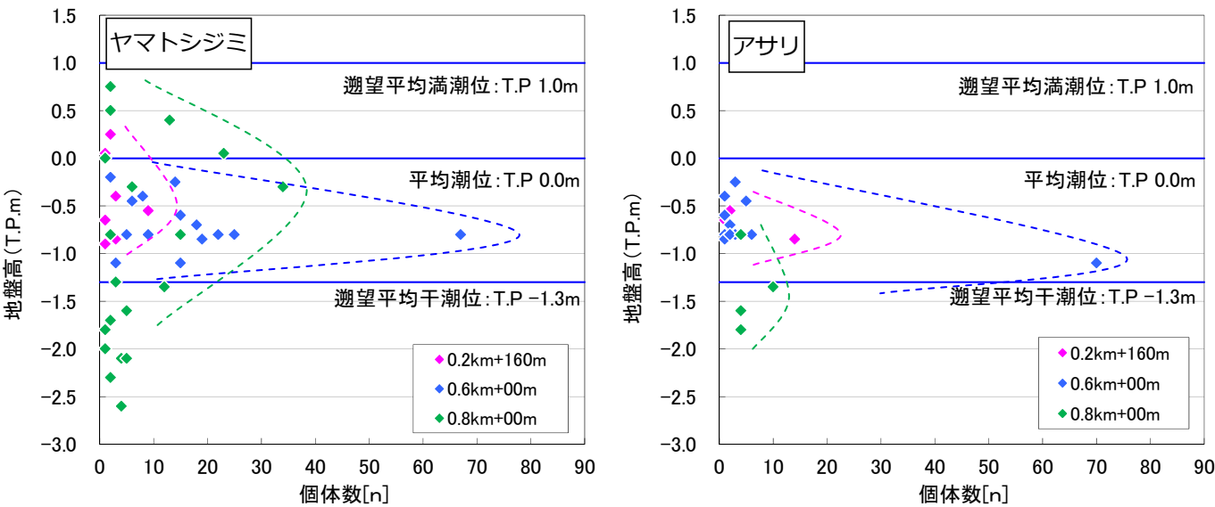
図ー 側線別にみたヤマトシジミ、アサリの地盤高分布
