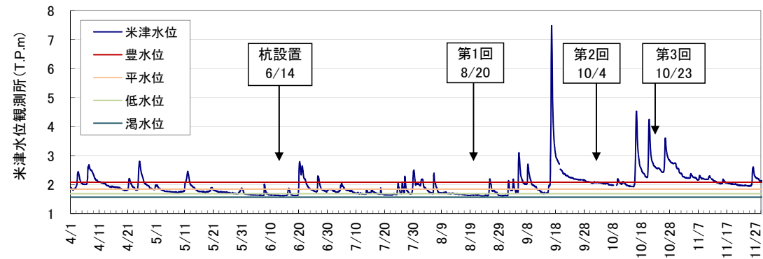
図- H25 年米津時間水位とリング調査実施状況
