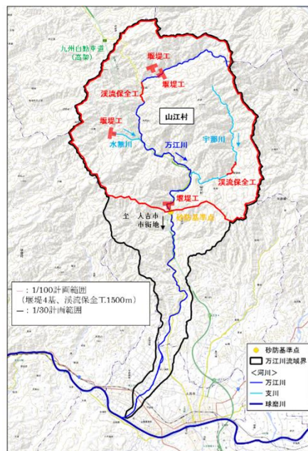
土砂・洪水氾濫対策の施設配置図
