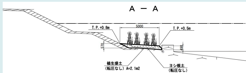
標準断面図(放水路左岸1.0-1.2k)
