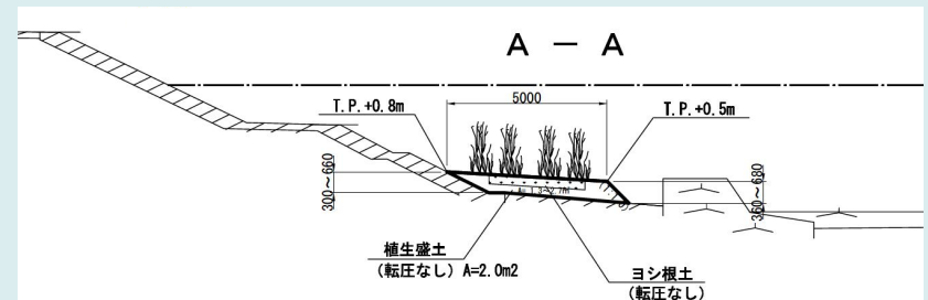
標準断面図(放水路左岸1.3-1.8k)
