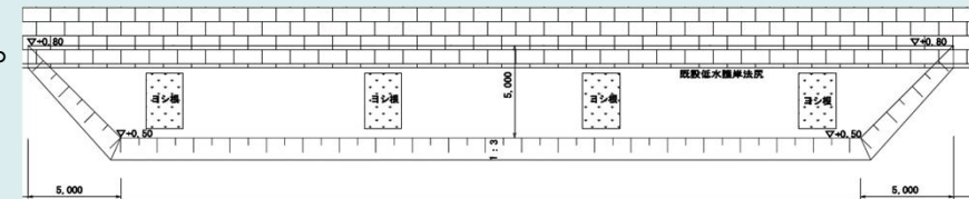
造成基盤ブロックの標準平面図 (放水路左岸1.3-1.8k)
