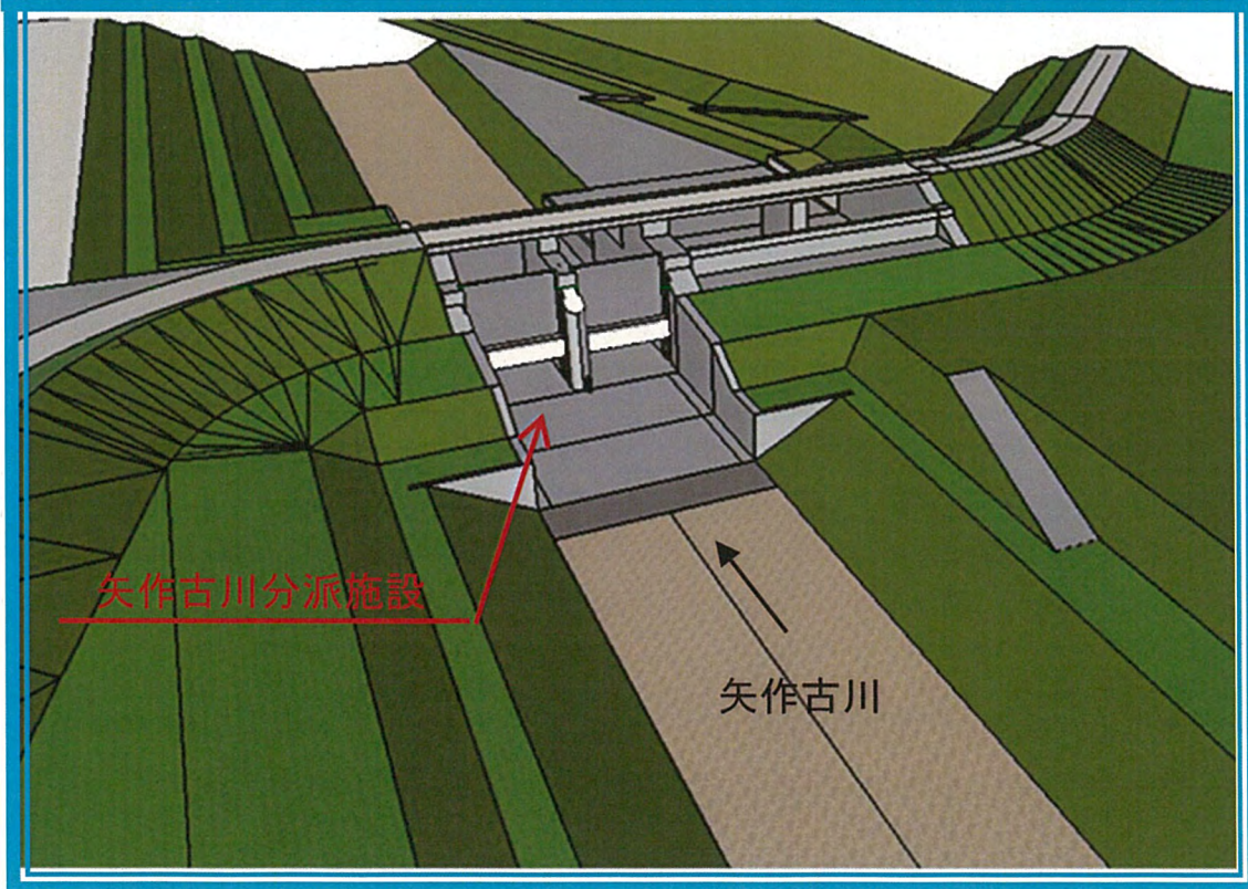
■ 矢作古川上流からみた分派施設の完成イメージ図
