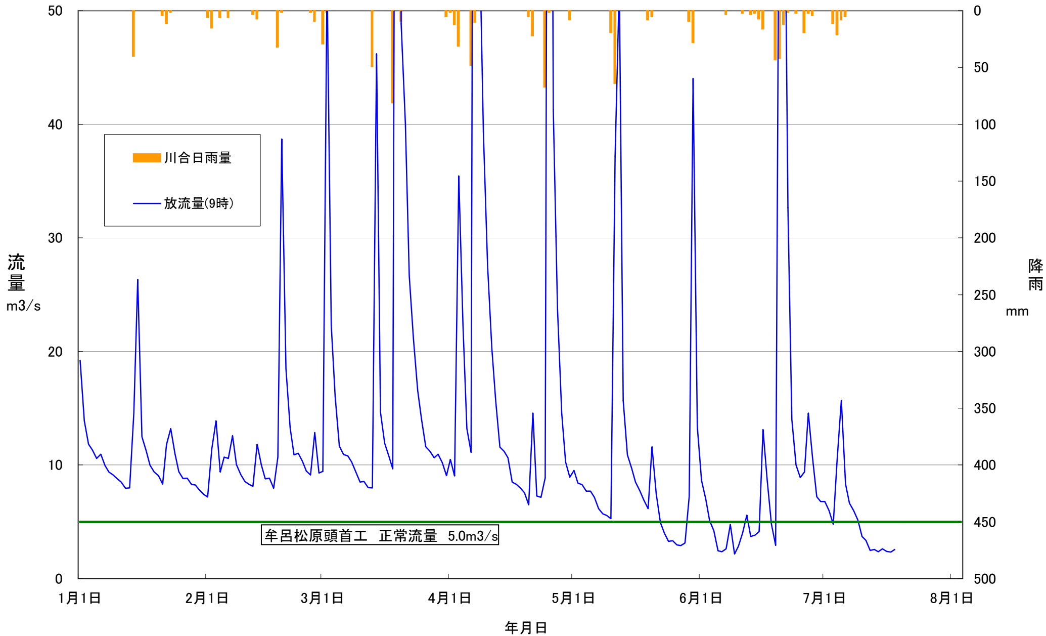
平成25年豊川河川流量（牟呂松原頭首工直下流放流量・速報値）
