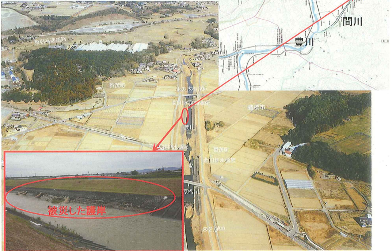
写真-1 被災箇所位置と被災状況
