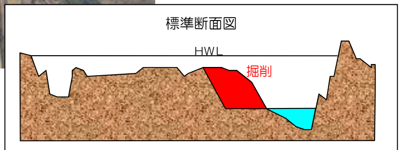
■掘削イメージ図
