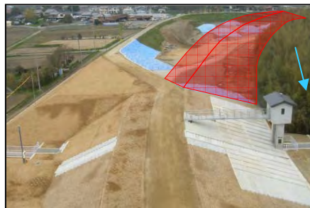
大村地区堤防整備(豊橋市)
