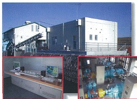
操作室内部 小坂井排水機場ポンプ設備
