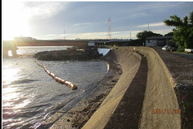
豊川 & 放水路と合流右岸先方護岸工事現場
