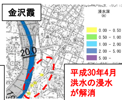
仮に整備計画(河道改修+設楽ダム)が 完成していた場合の効果
