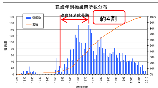
東海4県の市町村管理橋梁の現状(橋長1.5m以上) H24.4.1現在
