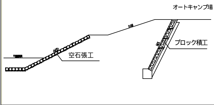
護岸工構造図
