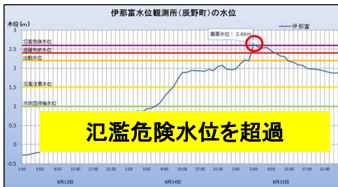
伊那富水位観測所の水位
