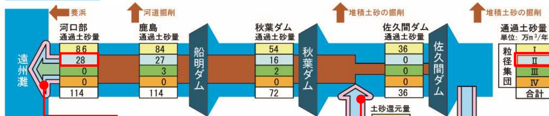
河口テラスの回復のイメージ
