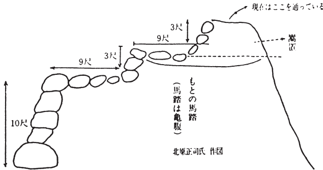
図一 8 石川除構造図
