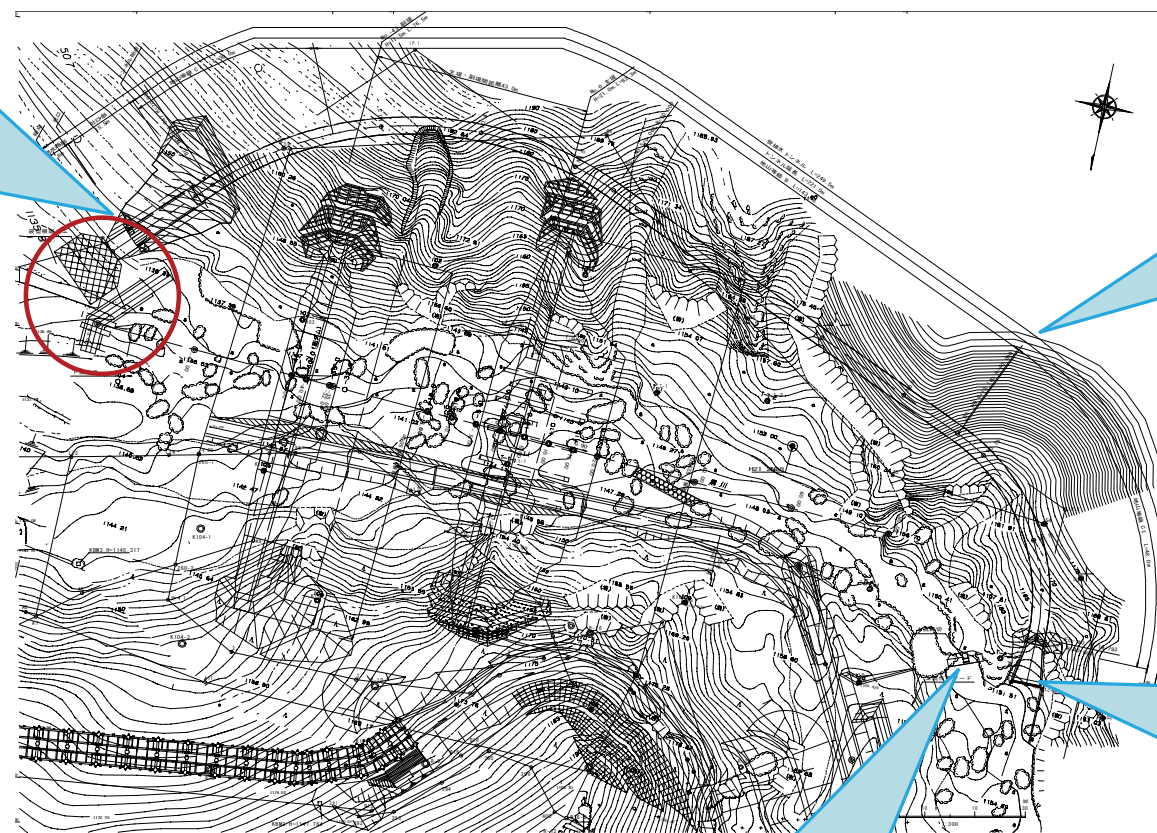
川の流れをトンネルに導くためのコンクリートの擁壁(締切)です
