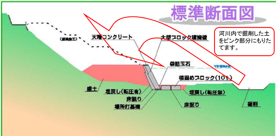
掘削した土を再利用し、擁壁背面を盛り立てます。(下流側)
