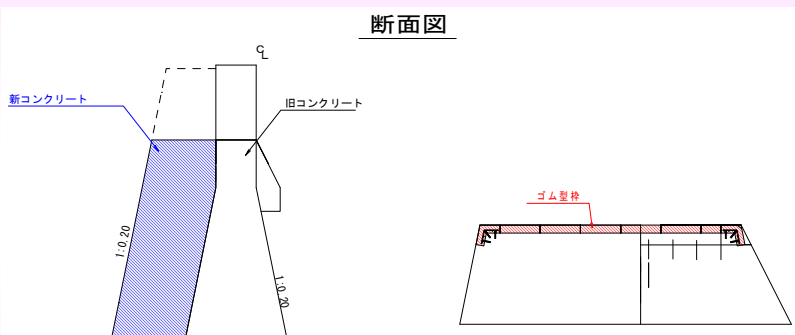
釜沢砂防えん堤
