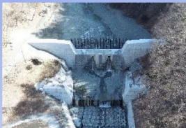
鋼製スリット 据付完了 (上流側より撮影)
