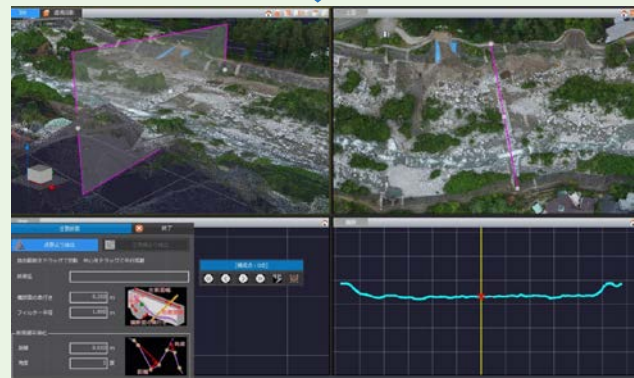
断面形状や施工量等を容易に確認できる
