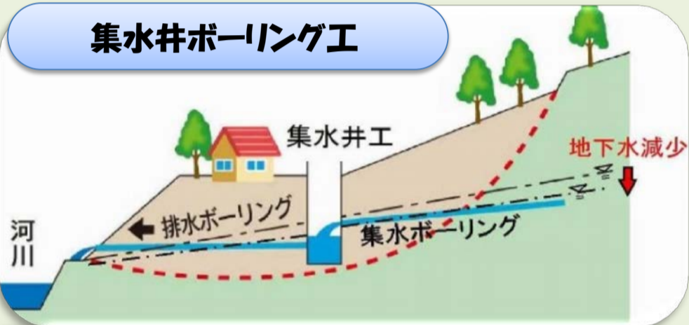
集水井
