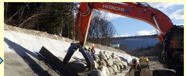
② 令和4年12月～ 護岸に巨石(現地発生材)を設置
