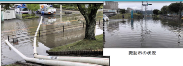
長野県諏訪市での排水作業（天竜川上流の排水ポンプ車 R3.8/15～16）
