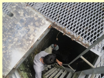
入谷地区地すべり対策事業の 集水井を見学
