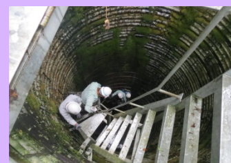
▲入谷地区地すべり 集水井の中へ
