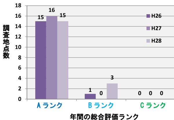
「利用しやすい水質の確保」の視点のランク別地点数
