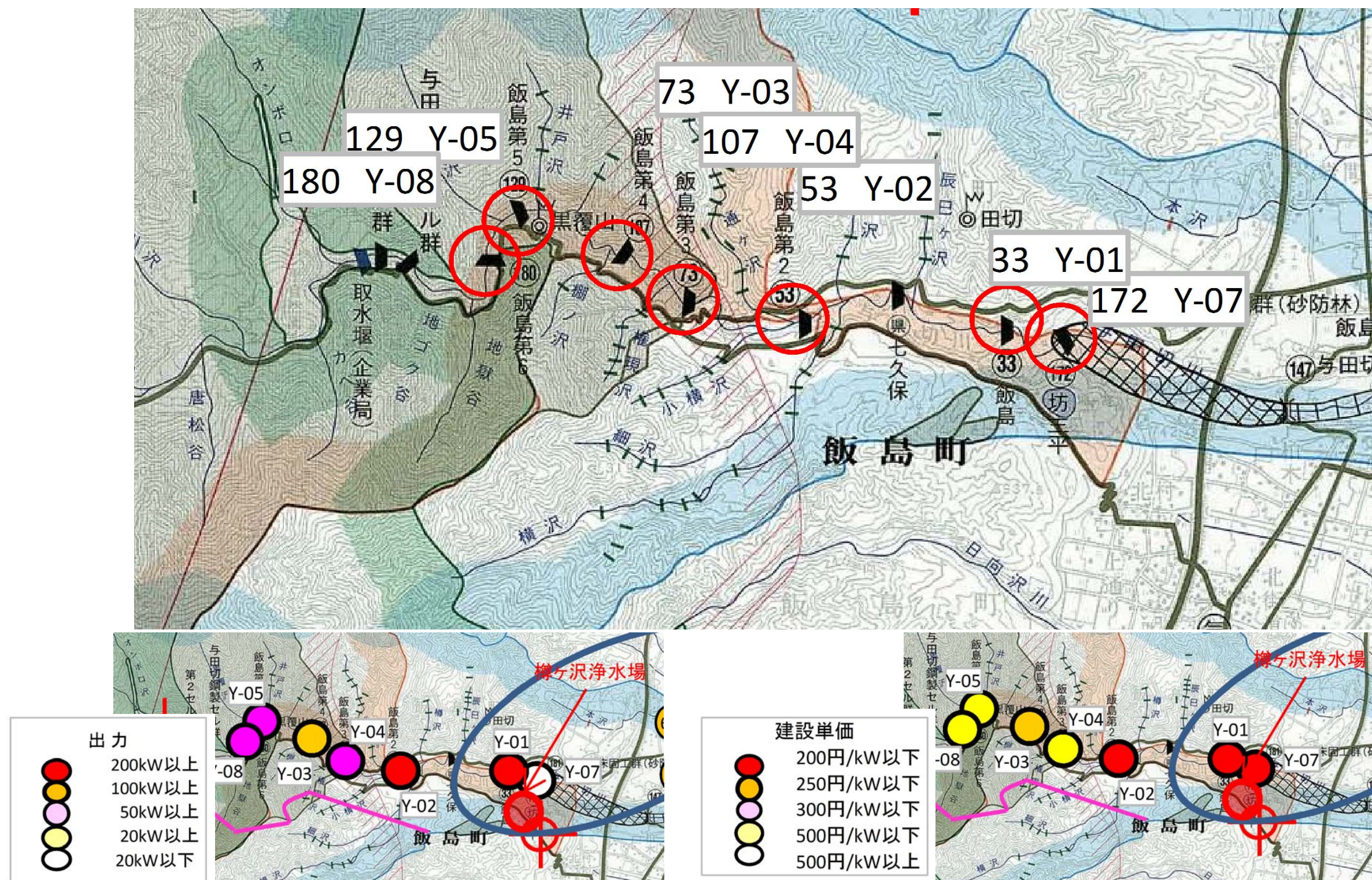
図 1 砂防施設位置図
