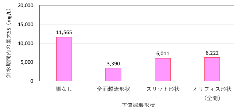
構造ごとの最大SSの比較
