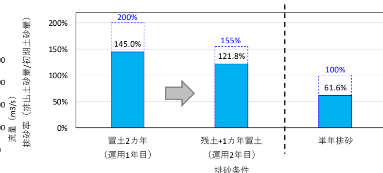
通水後の条件ごとの排砂率の比較
