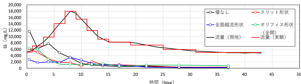
ストックヤード内土砂の排出状況の比較
