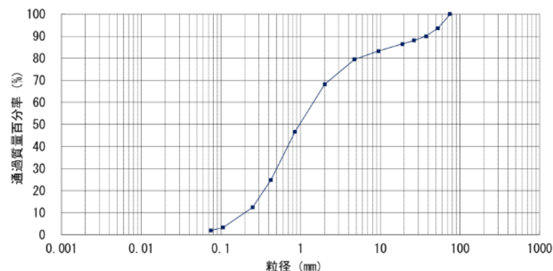
平成28年度置土試験工事 粒径加積曲線
