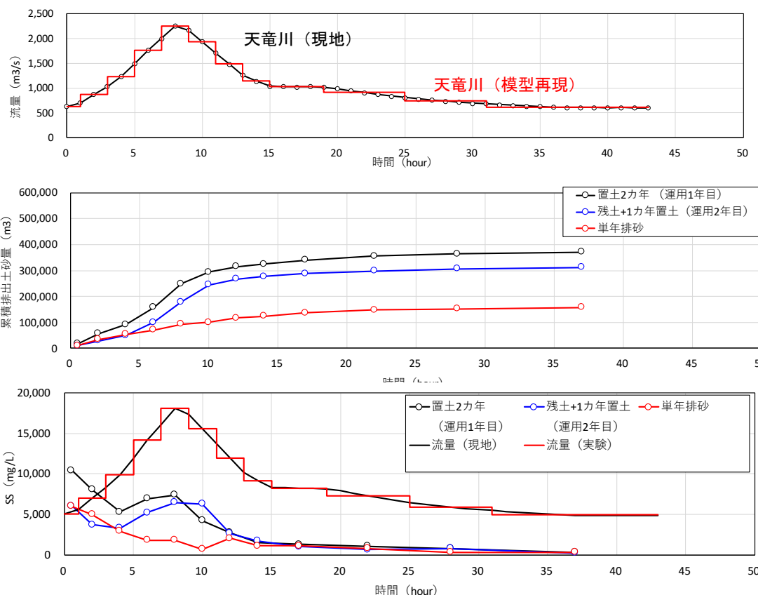
ストックヤード内土砂の排出状況の比較 (暫定値)
