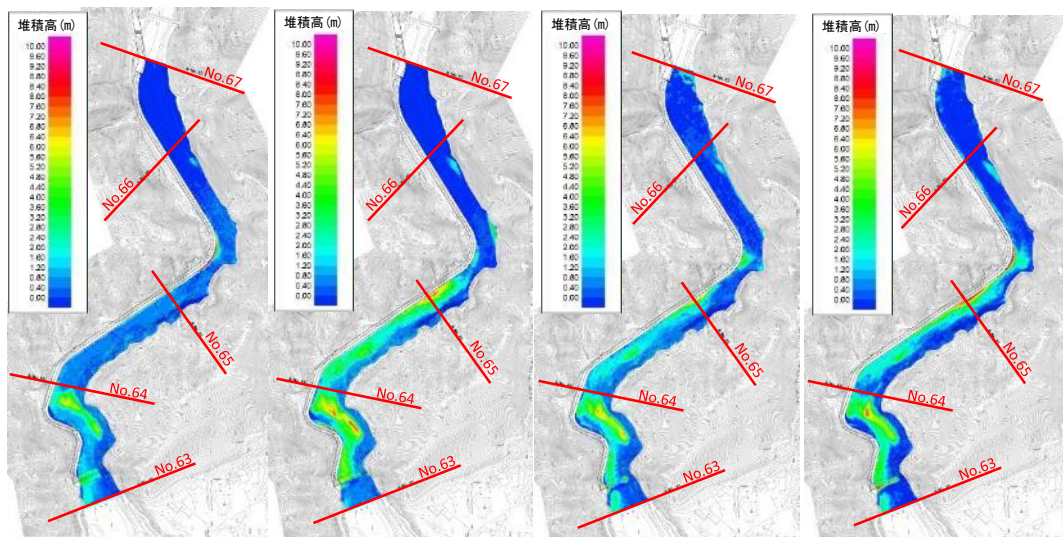
①堰なし ②全面越流形式 ③スリット形式 ④オリフィス形式 (全開)
