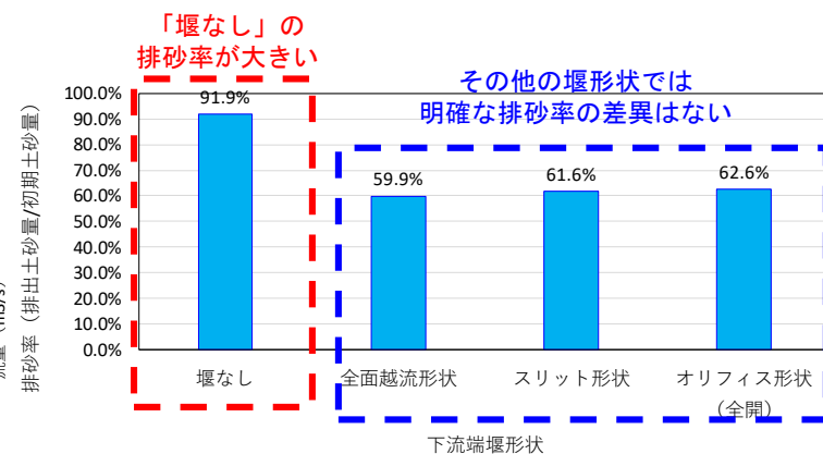
通水後の構造ごとの排砂率の比較
