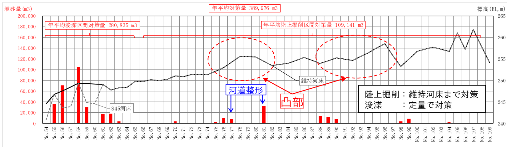
新たに検討した維持河床(凸部掘削なし)と地点毎の堆砂量
