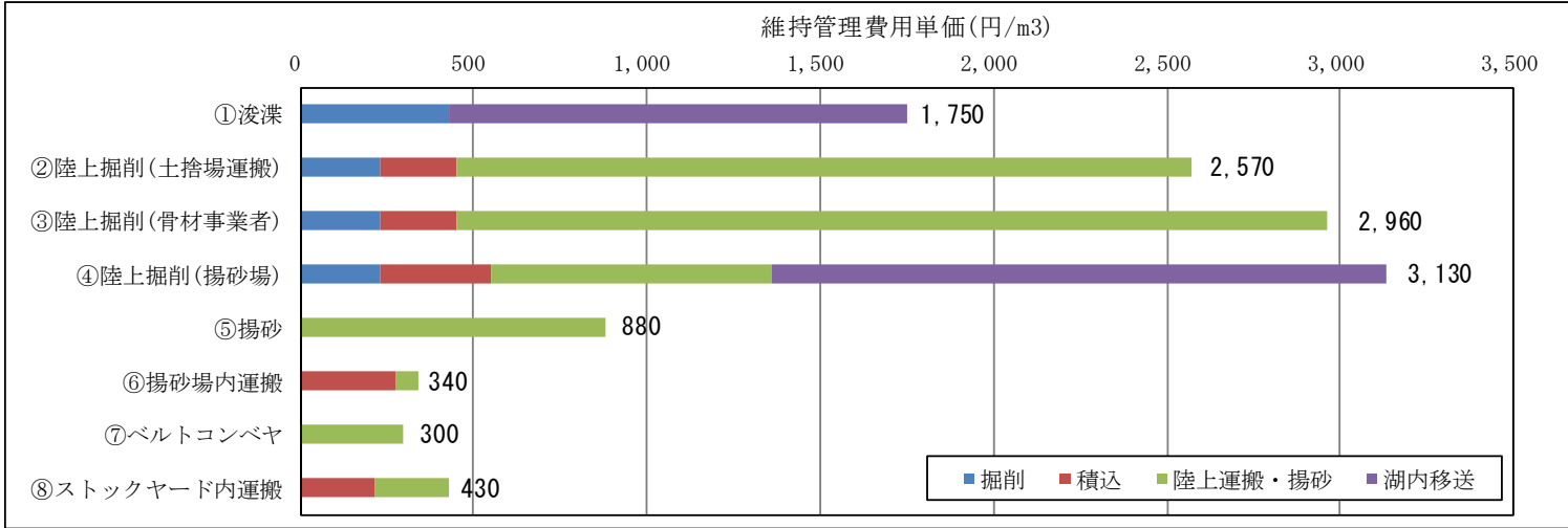
維持管理費用単価の内訳（対策土砂量44万m 3 /年）
