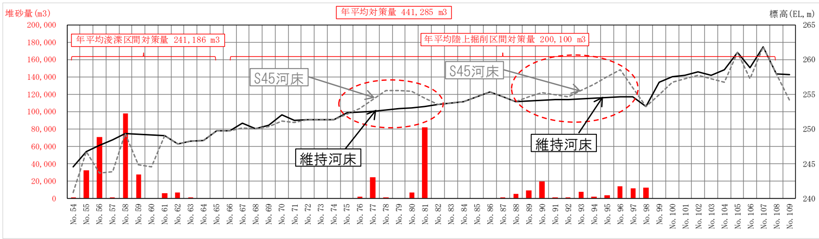
断面毎の対策土砂量（100年間平均値）
