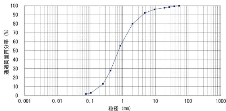
平成29年度置土試験工事 粒径加積曲線
