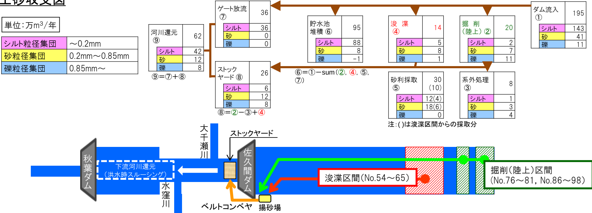
土砂収支図
