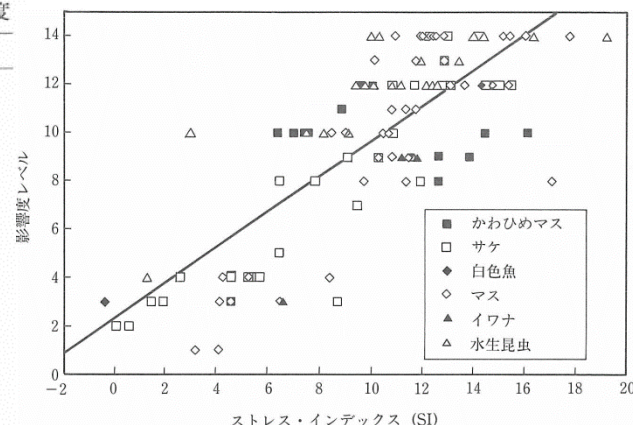
図-3 ストレス・インデックス (SI) と生態系への影響度レベルの関係
