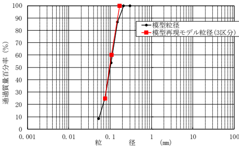
模型粒径を3粒径区分で再現
