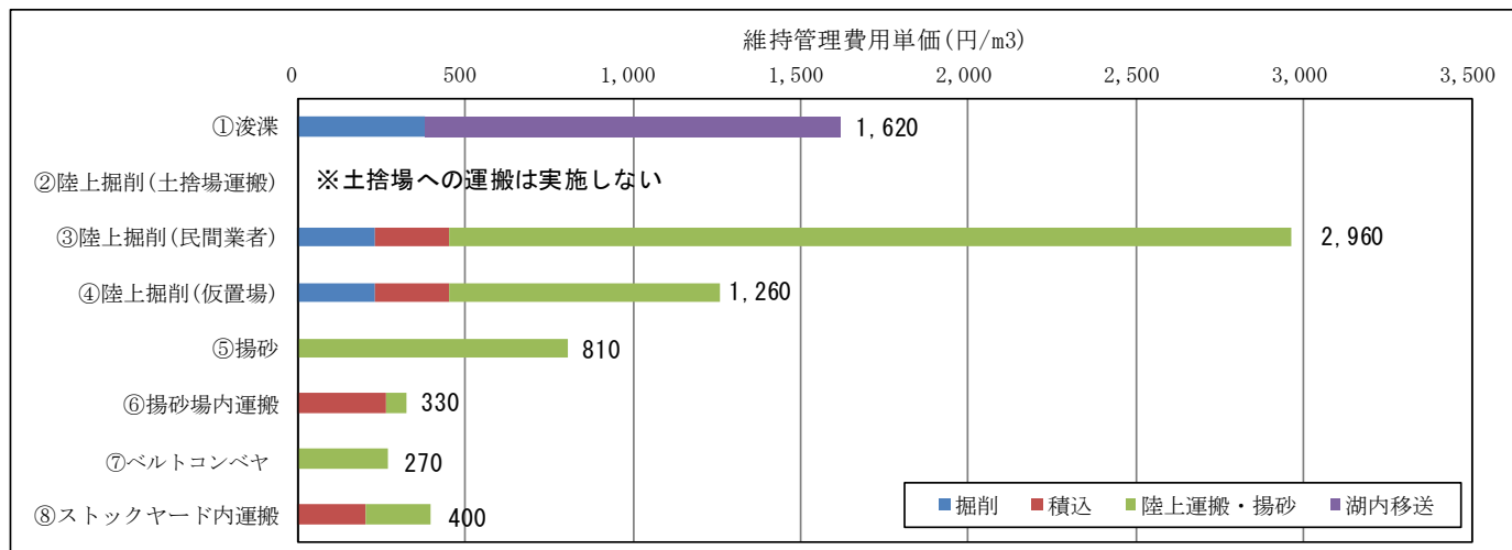
維持管理費用単価（対策土砂量39万m 3 /年，今回検討結果）
