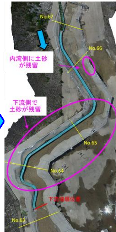
年平均洪水の通水後
