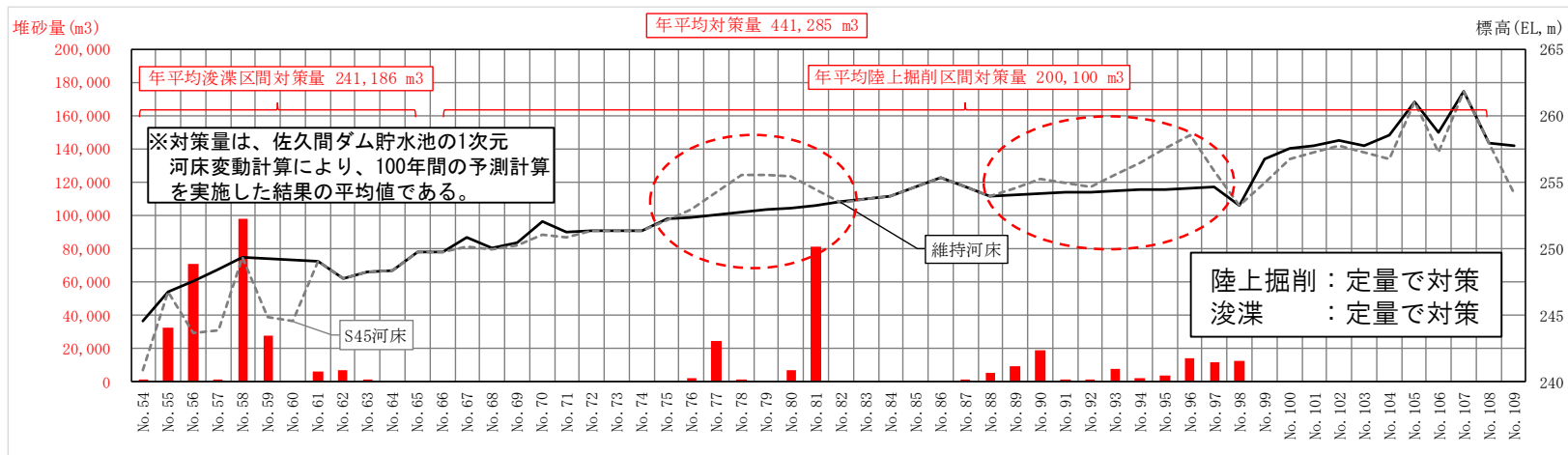
第3回委員会で提示した維持河床(凸部掘削あり)と地点毎の堆砂量
