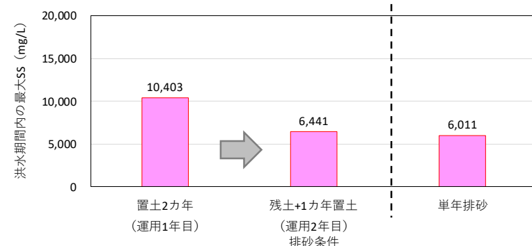
条件ごとの最大SSの比較
