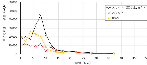
流入土砂条件 (実験結果による時間あたり排砂量)
