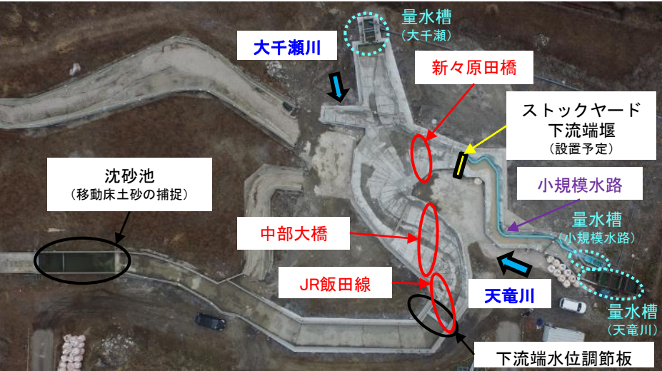
模型再現範囲
