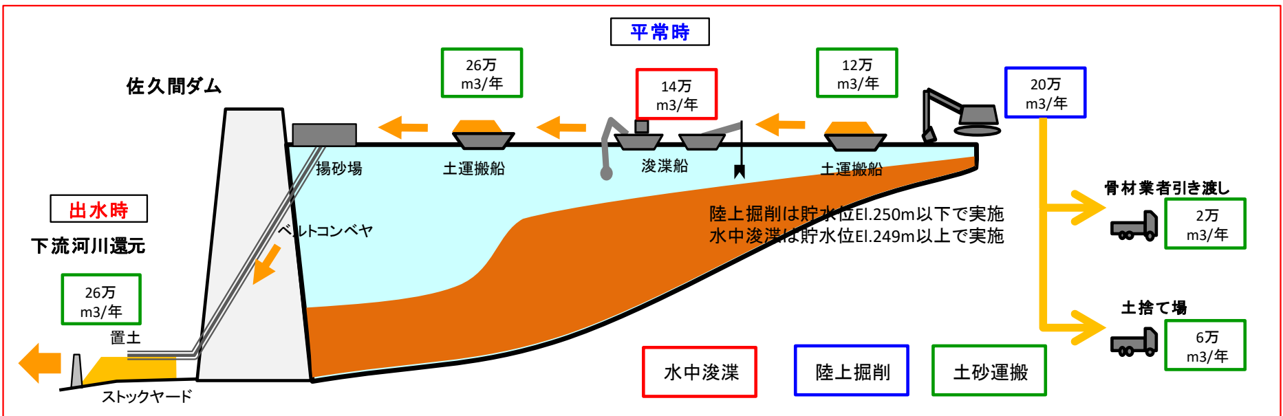
堆砂対策工法の構成
