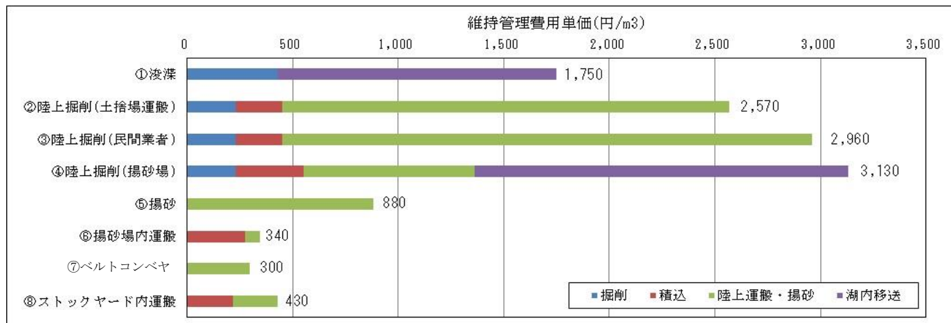
維持管理費用単価（対策土砂量44万m 3 /年※，第3回委員会提示）※44万m 3 のうち10万m 3 は民間活用
