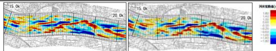
現状継続 排砂実施時 平面二次元河床変動計算による予測結果
