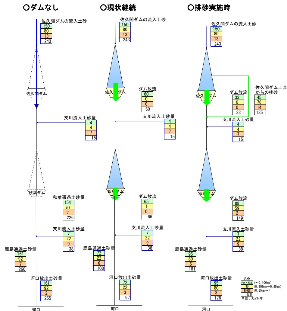
砂フラックス（砂礫）の予測結果（26か年の平均値）
