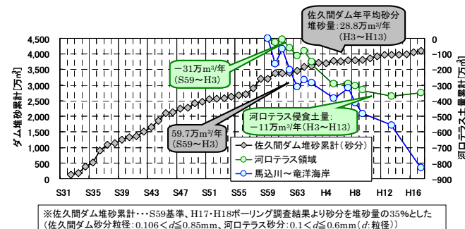
河口テラスボリュームの減少と佐久間ダム堆砂量との関係
