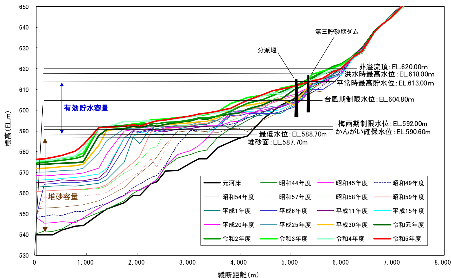
小渋ダム最深河床高の推移
