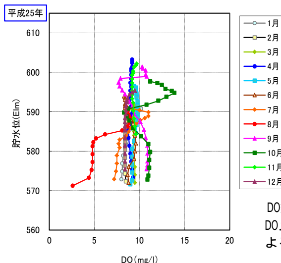
貯水池内のDO鉛直分布
