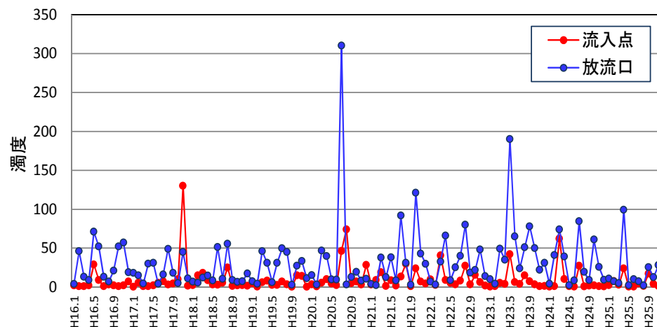
流入水と放流水の濁度の比較
