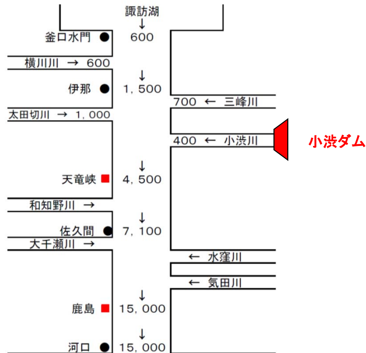
天竜川計画高水流量配分図
