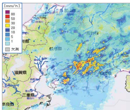
レーダ雨量 (6月30日23時30分)
