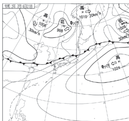
7月6日 21時00分 天気図 出典: 気象庁HP
