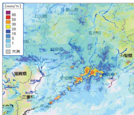
レーダ雨量 (7月6日20時20分)
