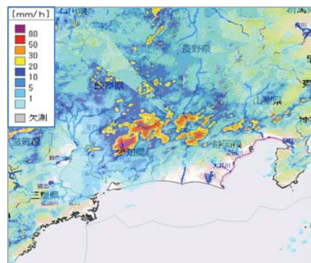
レーダ雨量 (7月8日4時40分)
