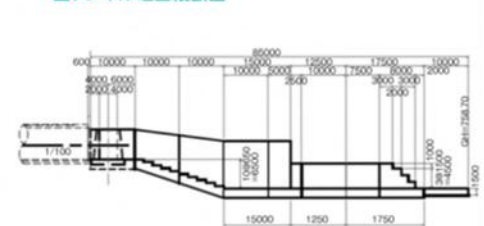
■トンネル吐口縦断面図
