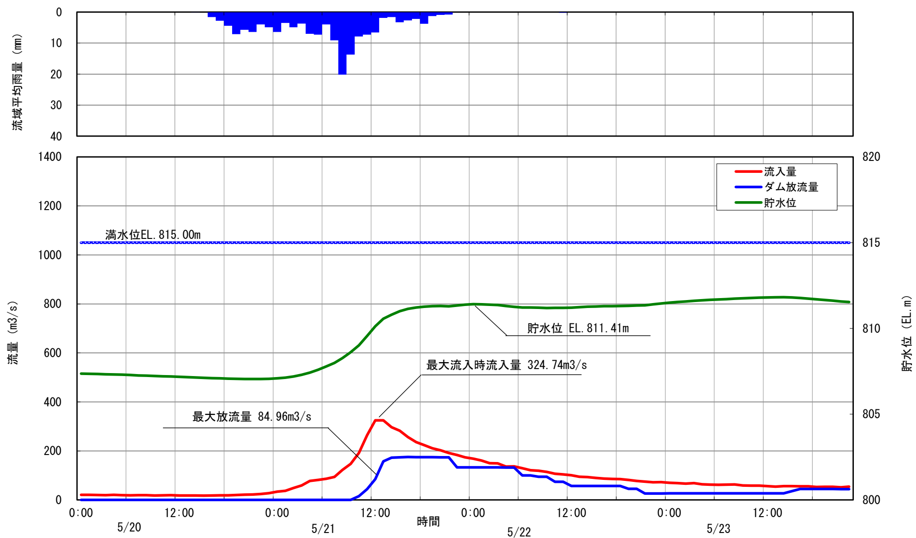
3 美和ダム洪水調節図 令和 3年5月21日洪水
