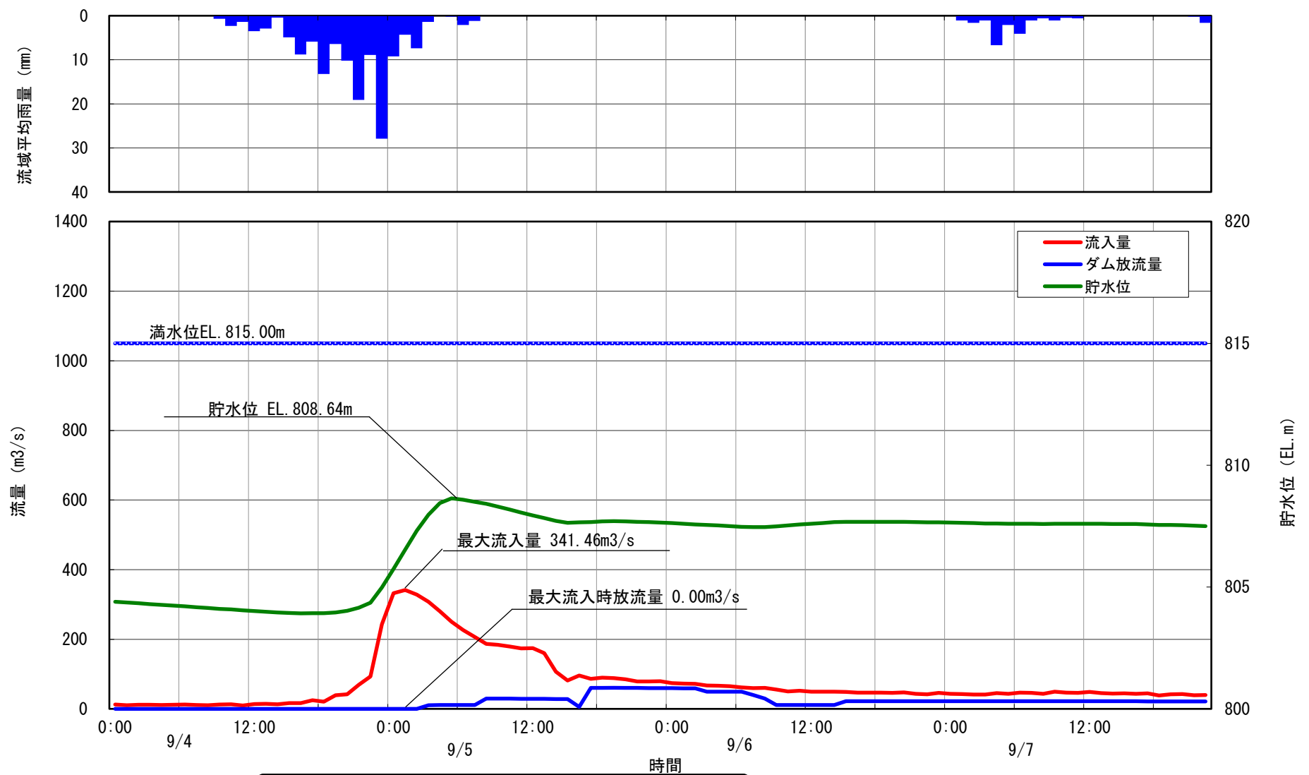
25 美和ダム洪水調節図 平成30年9月5日洪水
